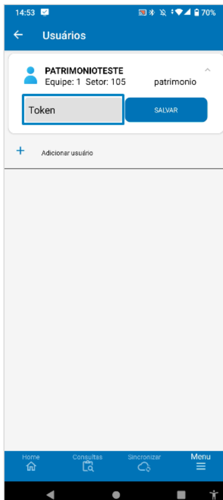
Figura 6: Token
